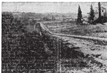
Aspecto de un sector de las obras de la «Urbanización MAS TRADER», en que se observa el creciente desarrollo de las mismas, apreciando el perfecto traslado de sus avenidas, bordillos tipo americano y las zanjas para la colocación de las conducciones de desagües
